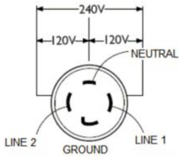
NEMA L14-30
